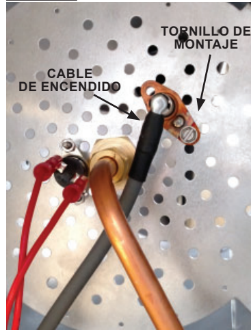
FIGURA 18 LA ANIELA SE DEBE COLOCAR ENTRE EL ENCENDEDOR Y LA PLACA DEL QUEMADOR
